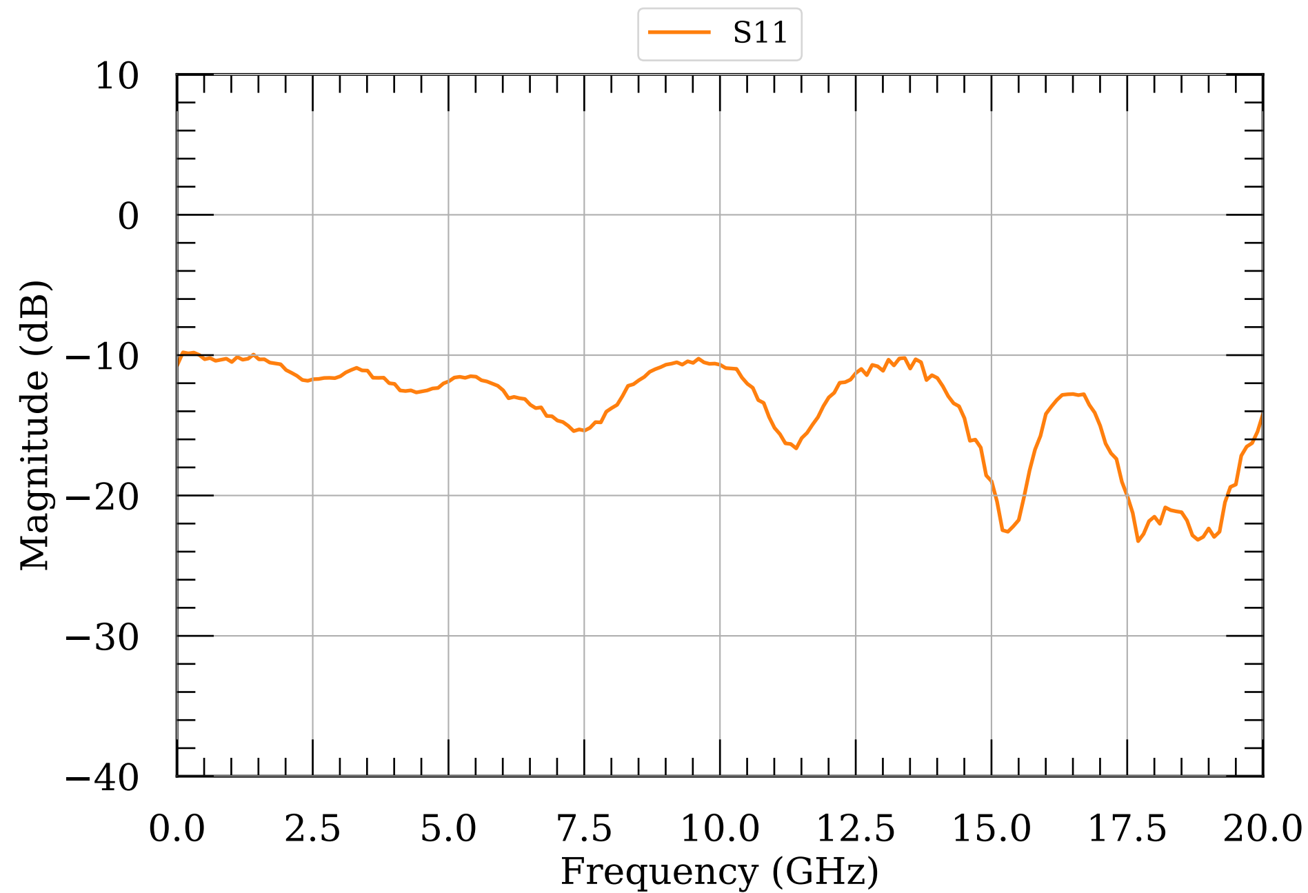
LNA S-params module067
